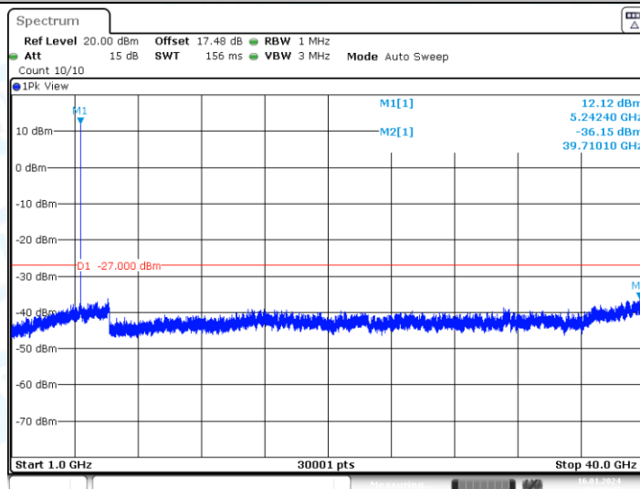
11N20MIMO_Ant1_5240_1000~40000
