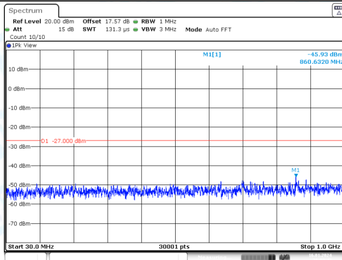
11N20MIMO_Ant2_5240_30~1000
