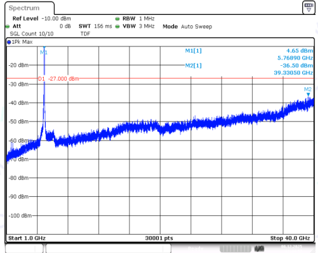
11AC80SISO-Ant1-5775-1000~40000-PASS
