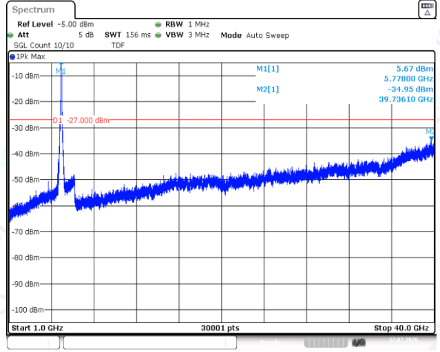
11AC80SISO-Ant1-5775-1000~40000-PASS
