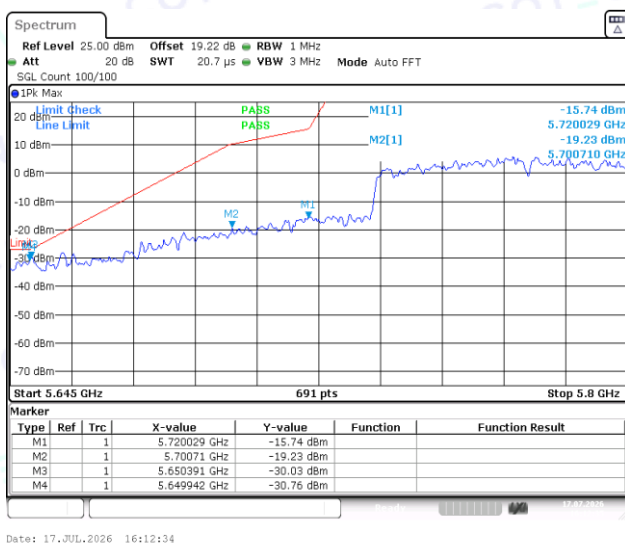
11AC80SISO-Ant1-5775-PASS
