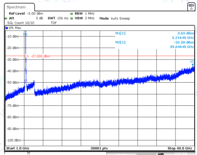
11AC80SISO-Ant1-5210-1000~40000-PASS
