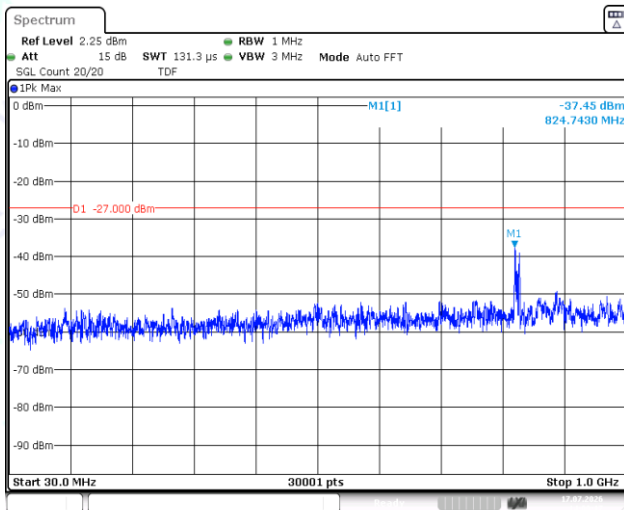
11A-Ant1-5745-30~1000-PASS
