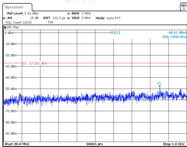
11A-Ant1-5200-30~1000-PASS
