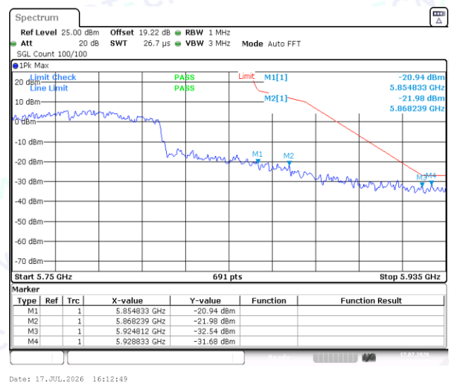
11AC80SISO-Ant1-5775-PASS
