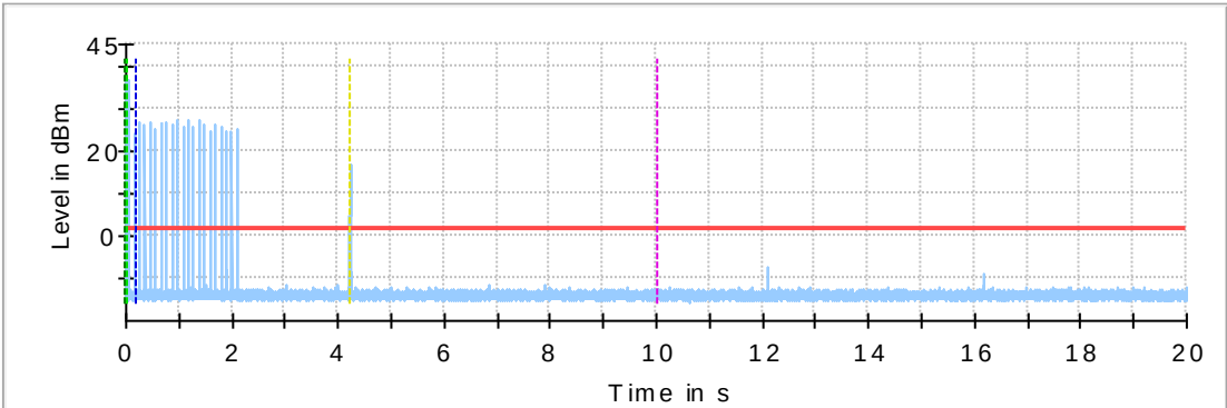
802.11a 5260MHz
