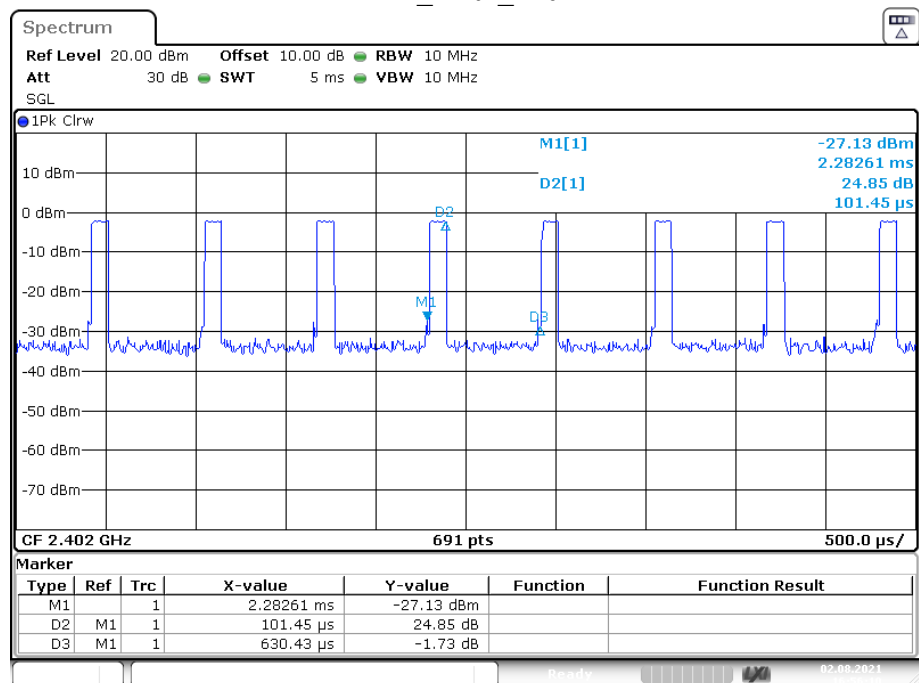
BLE_Ant1_2402
