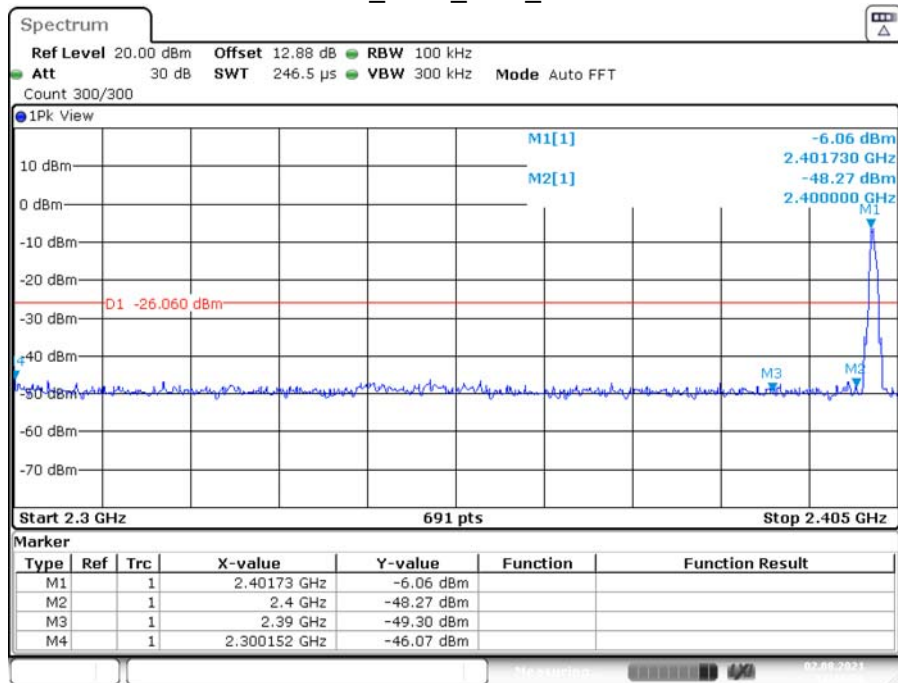
BLE_Ant1_Low_2402
