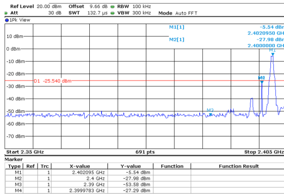
Figure 5: Band Edge
