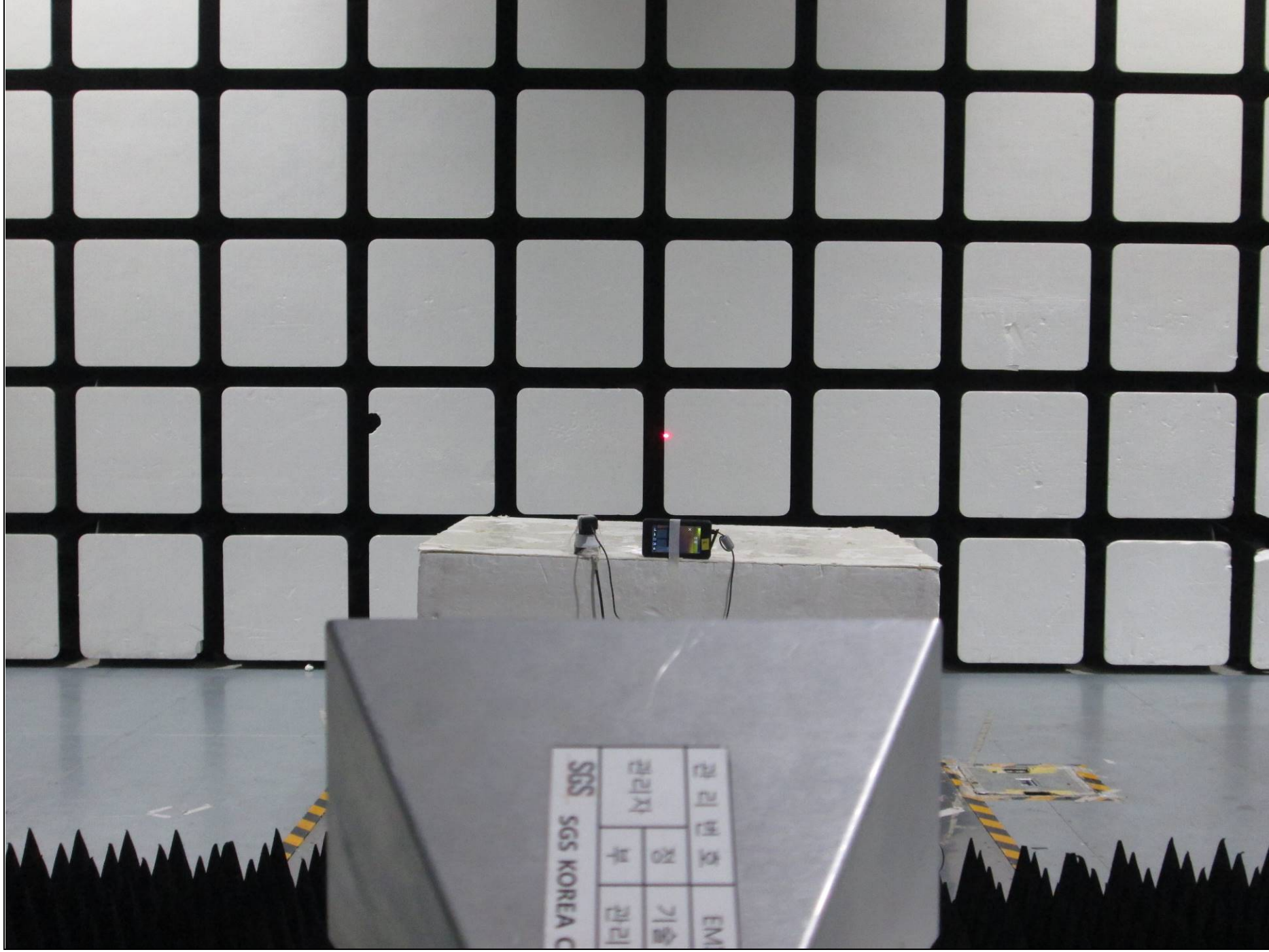
RE(Above 1 GHz)_Rear
