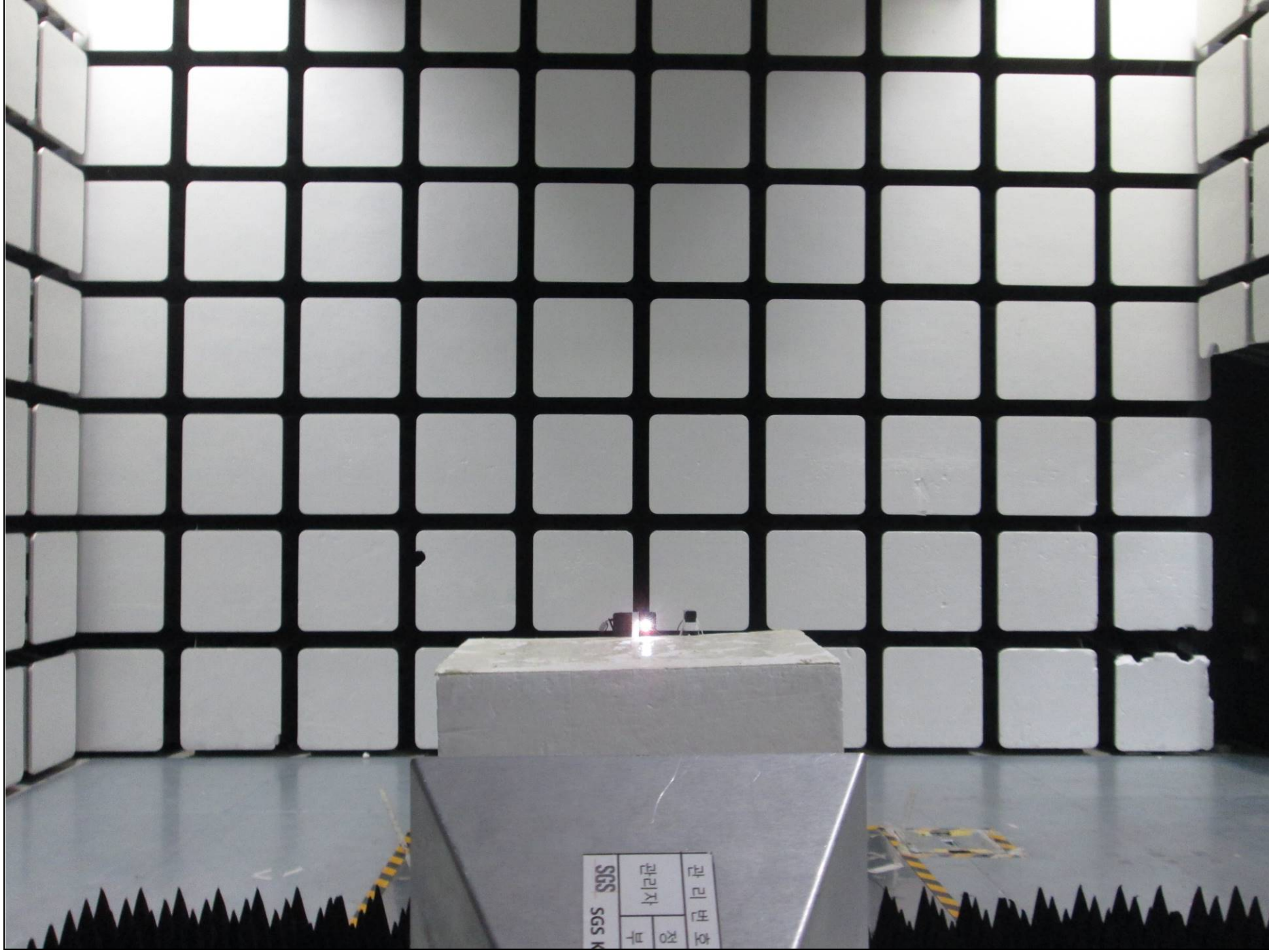
RE(Above 1 GHz)_Front
