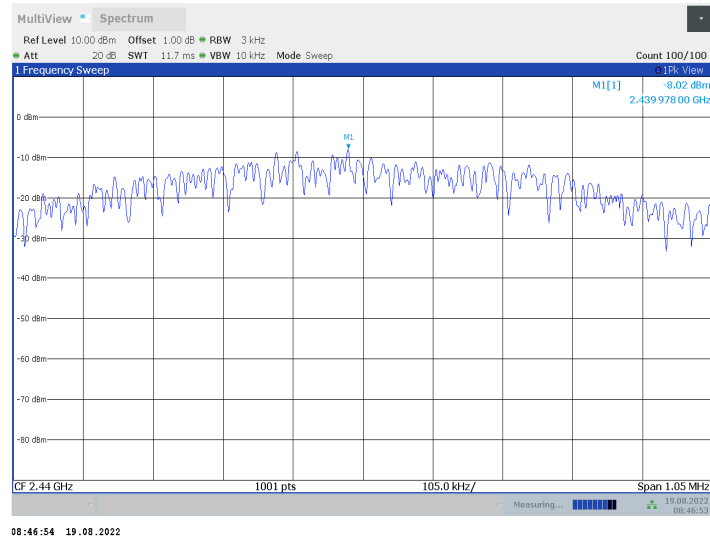
BLE_1M_Ant2_2440
