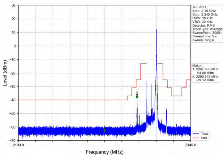
Band30_10MHz_16QAM_MCH_2310MHz_RB_1_0_NTNV
