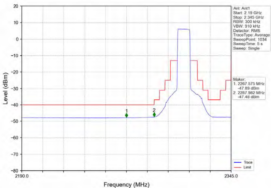
Band30_10MHz_64QAM_MCH_2310MHz_RB_1_49_NTNV
