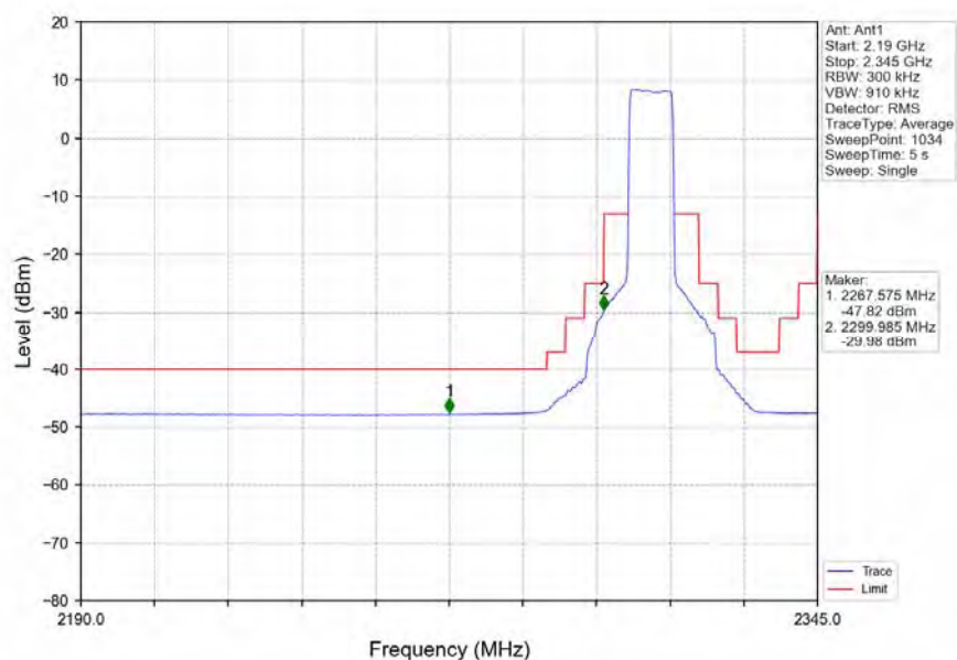
Band30_10MHz_QPSK_MCH_2310MHz_RB_1_49_NTNV
