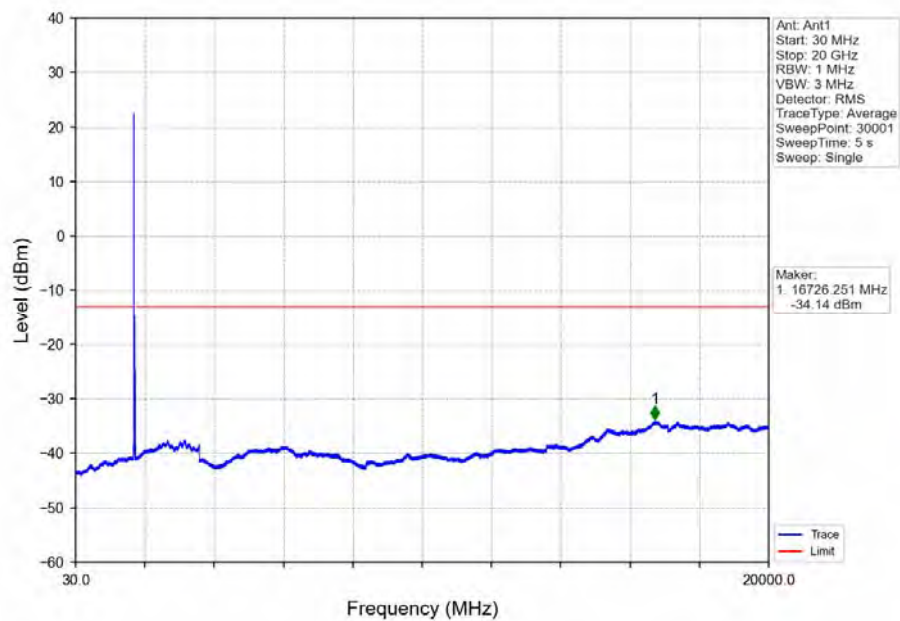
Band4_20MHz_QPSK_LCH_1720MHz_RB_1_0_NTNV
