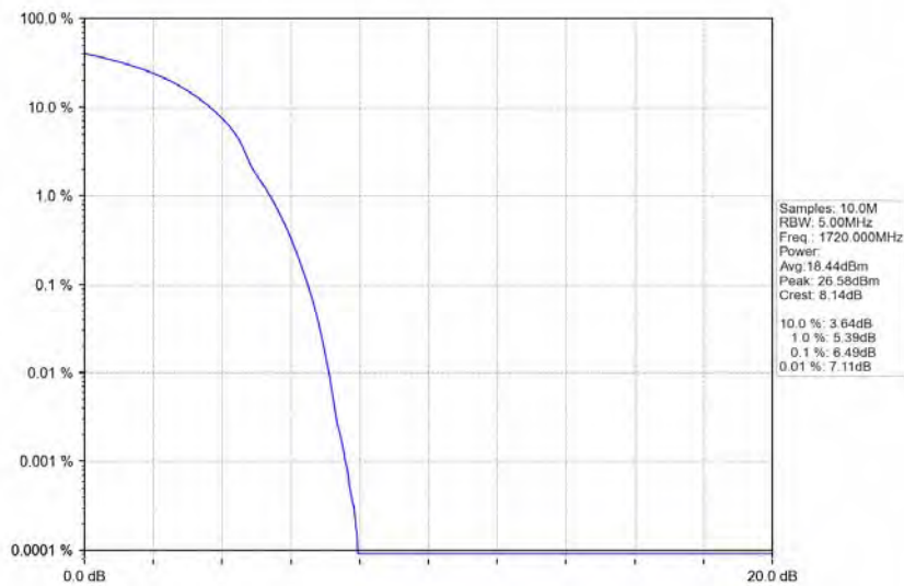
Band4_20MHz_QPSK_LCH_1720MHz_RB_100_0_NTNV
