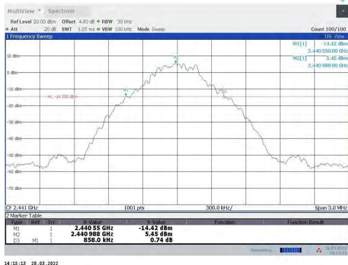
DH5 Ant 2 2441
