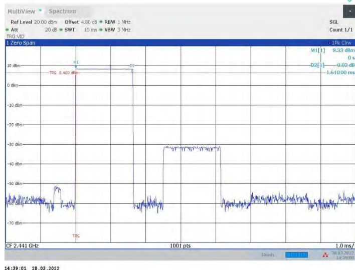
DH3_Ant 2_Hop
