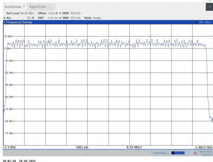
2DH5_Ant 2_Hop
