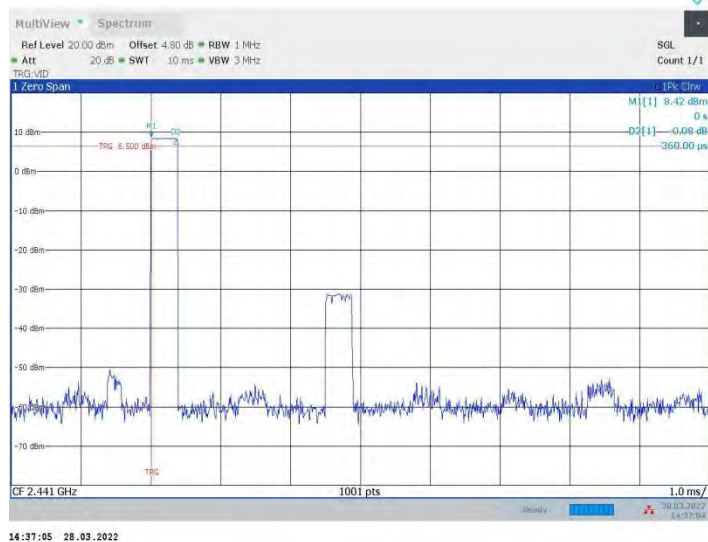
DH3_Ant 2_Hop
