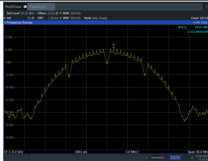
11B_Ant1_2412_0~Reference
