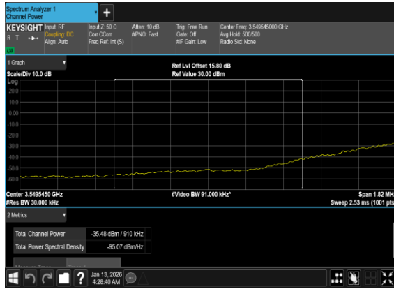
N77(90M)_DFT-s- OFDM_QPSK_Edge_1RB_Left_Low_CH_CHP_PASS
