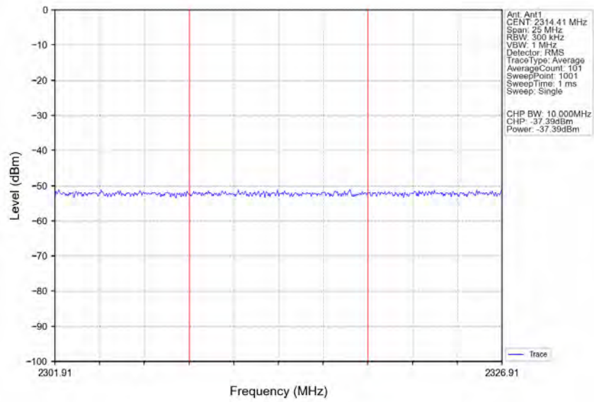
n30_15kHz_SISO_NTNV_10MHz_CP-OFDM_256_QAM_2310MHz_Inner_1RB_Right_Ant1
