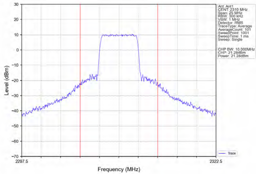
n30_15kHz_SISO_NTNV_10MHz_CP-OFDM QPSK 2310MHz_Inner_Full_Ant1
