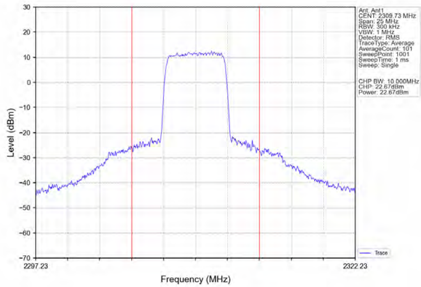
n30_15kHz_SISO_NTNV_10MHz_DFT-s-OFDM QPSK 2310MHz_Inner_Full_Ant1
