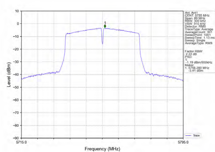
802.11ac(VHT40)_LCH_5755MHz_Ant1_NTNV
