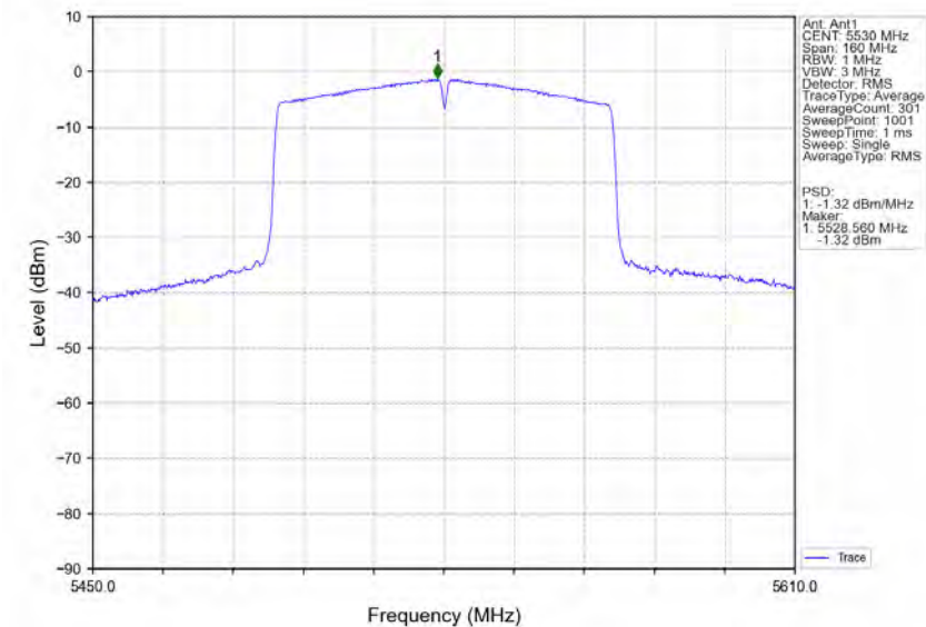
802.11ac(VHT80)_LCH_5530MHz_Ant1_NTNV
