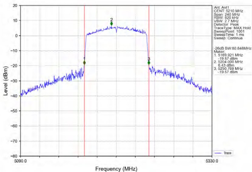
802.11ac(VHT80)_MCH_5210MHz_Ant1_NTNV
