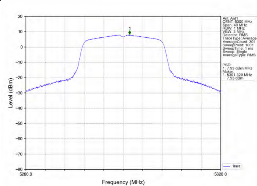
802.11a_MCH_5300MHz_Ant1_NTNV
