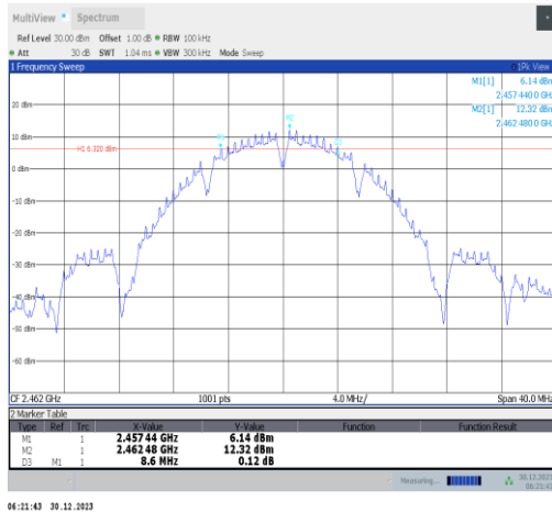
11b-Ant5-2462-PASS
