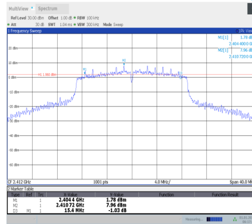
11n20ISO-Ant5-2412-PASS
