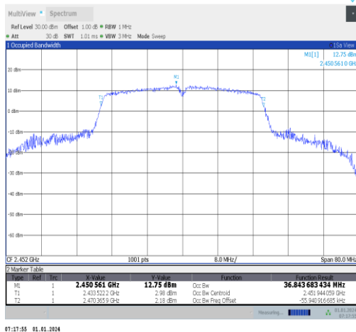
11n40ISO-Ant5-2452
