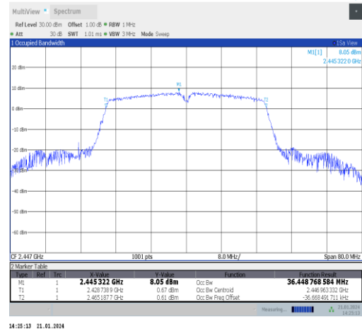
11n40ISO-Ant5-2447
