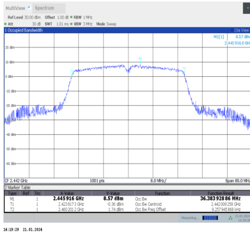
11n40ISO-Ant5-2442
