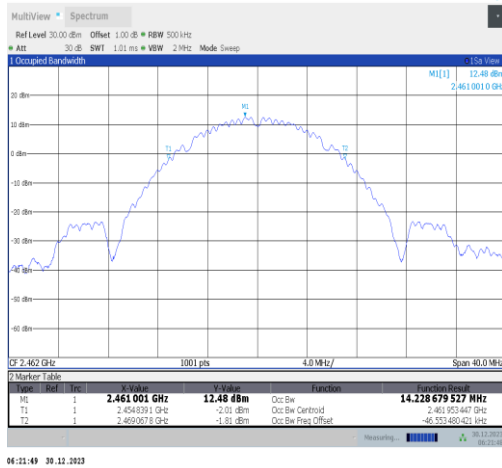
11b-Ant5-2462
