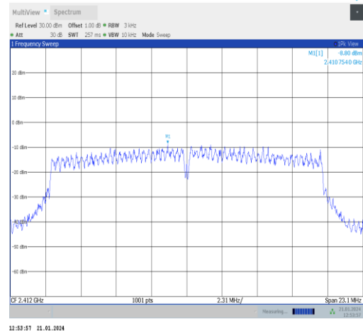
11n20ISO-Ant5-2412-PASS
