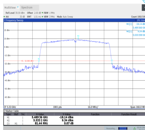
11ac80SISO-Ant5-5530
