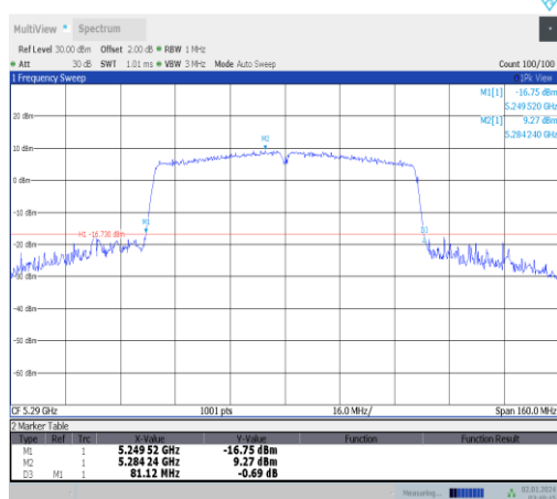
11ac80SISO-Ant5-5290
