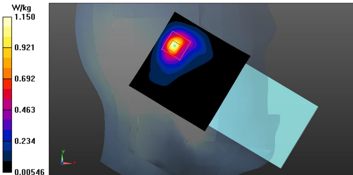
Fig.32 NR n77 Head
