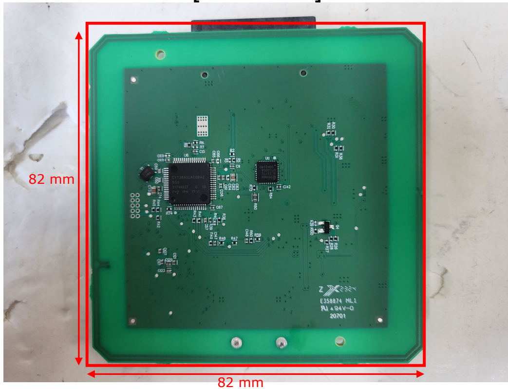
[NFC Antenna]
