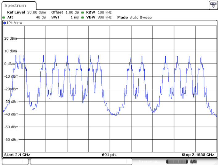
FSK Mode
