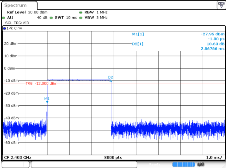
DH5_Ant1_Hop
