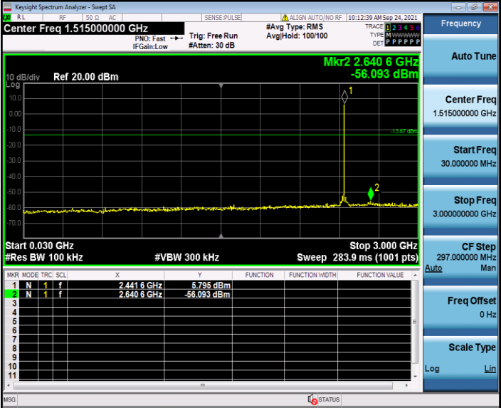
BLE 2440 30-3000
