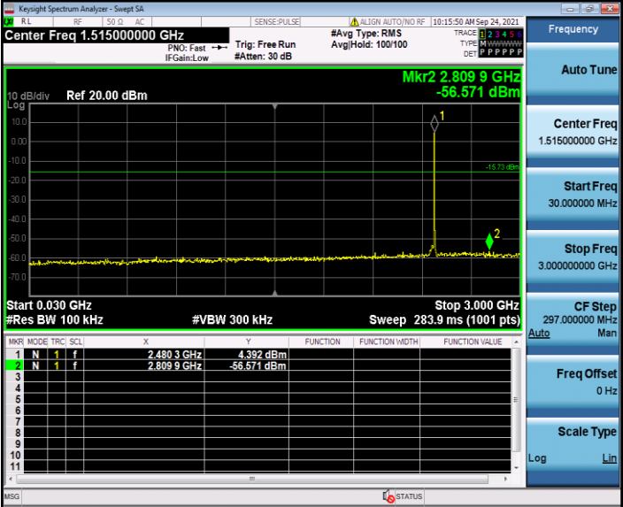
BLE_2480_30-3000
