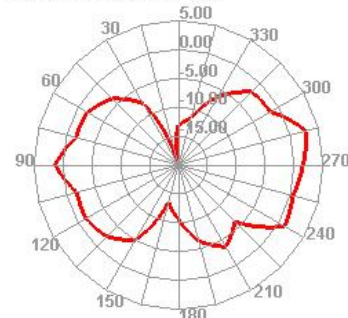
5100.000MHz E2
