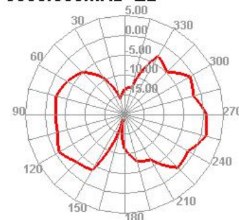
5850.000MHz E2
