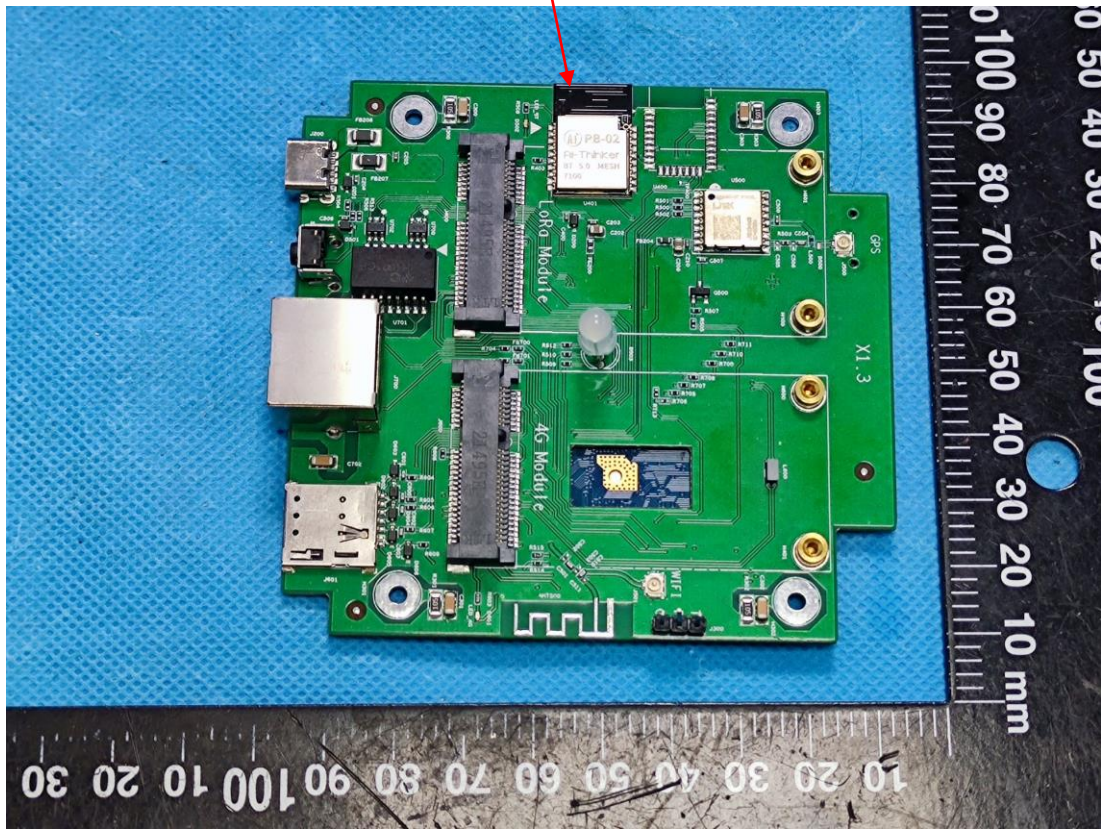
BLE Module
