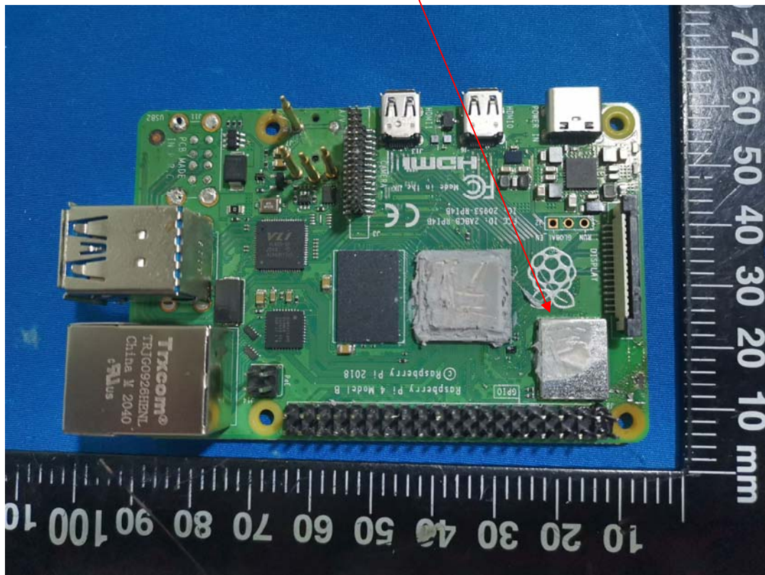
WiFi/BLE Module
