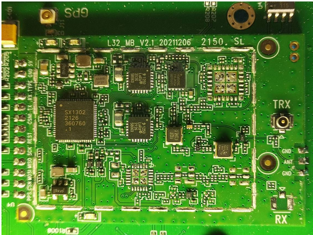
Lora Module
