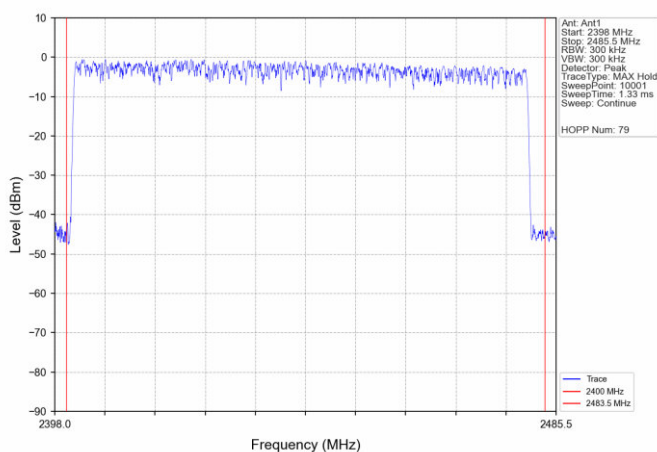
8DPSK_3DH5_HOPP_Ant1_NTNV
