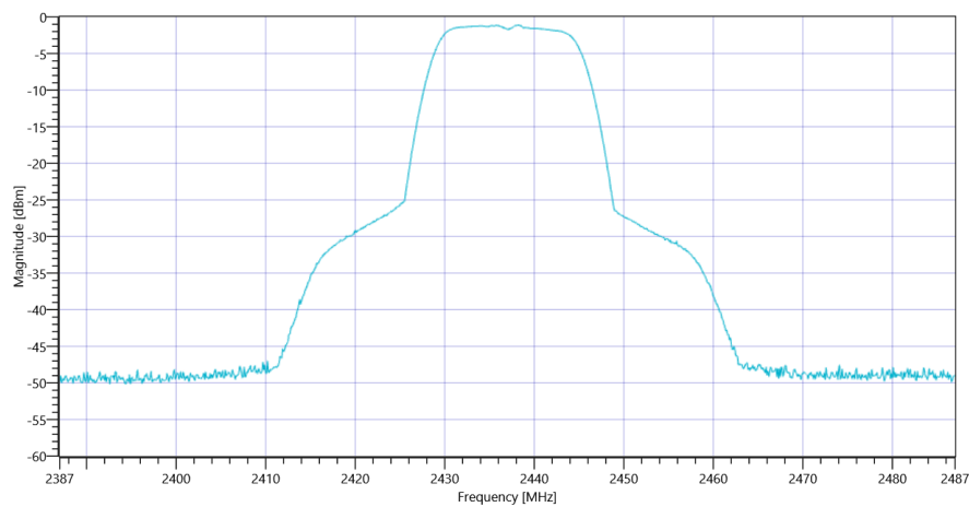
Plot_Common2G4 Peak OP 3MHz-3MHz ~ WLAN2G4 g-mode_07042021_140344.png
