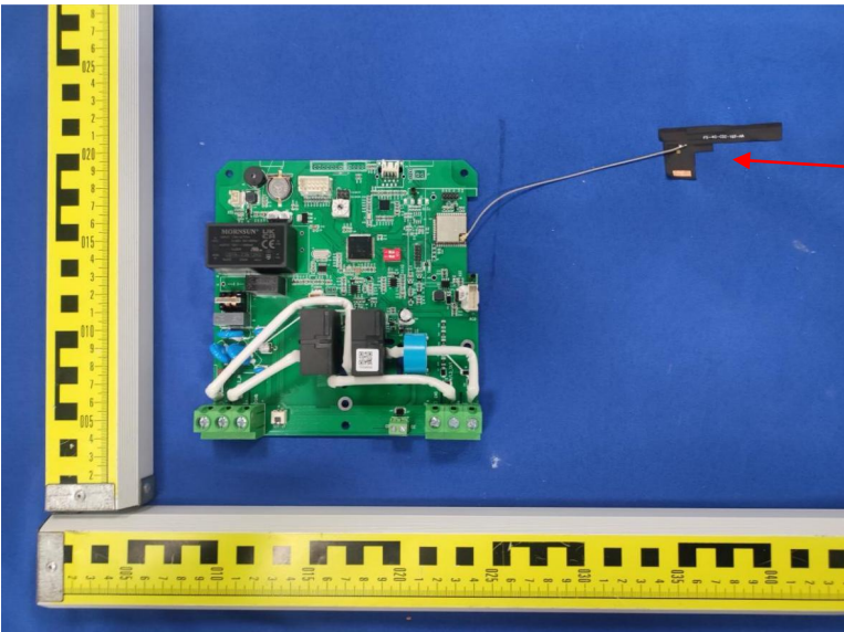
BT&WIFI Antenna
