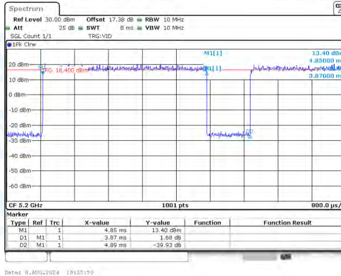
11AX20SISO_Ant1_5200
