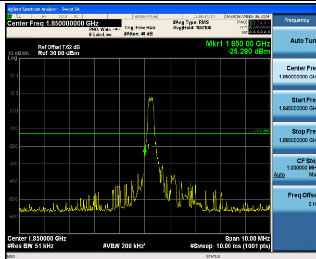
Band25-1.4MHz-QPSK-26047-1-0-Low--25.28-PASS
