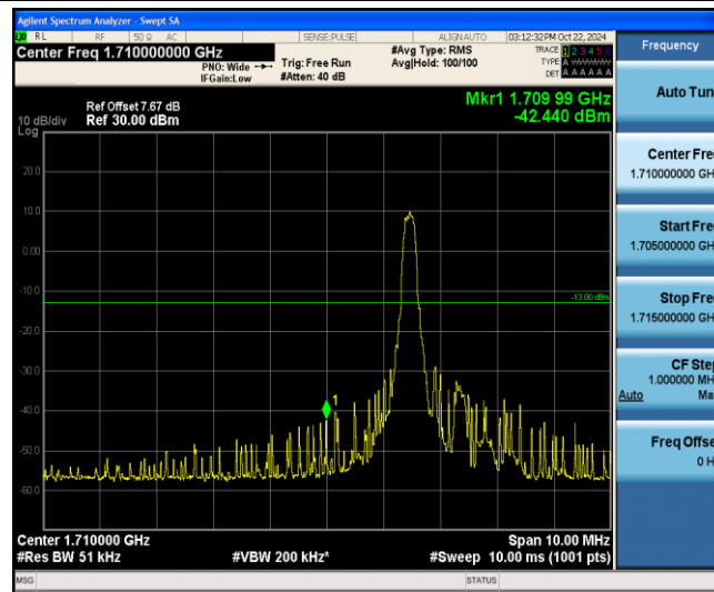
Band4-20MHz-QPSK-20050-1-0-Low--42.44-PASS
