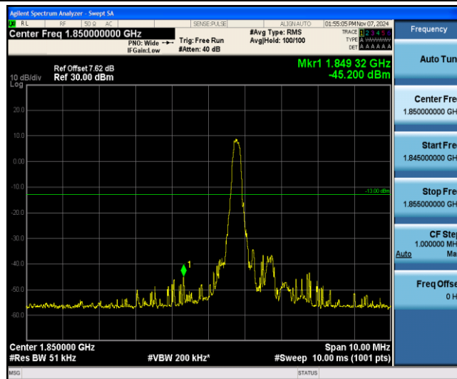
Band25-10MHz-QPSK-26090-1-0-Low--45.20-PASS
