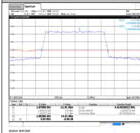
Band25-10MHz-16QAM-26365-50RB#0-PASS
