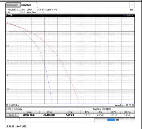
Band25-10MHz-16QAM-26365-50RB#0-PASS
