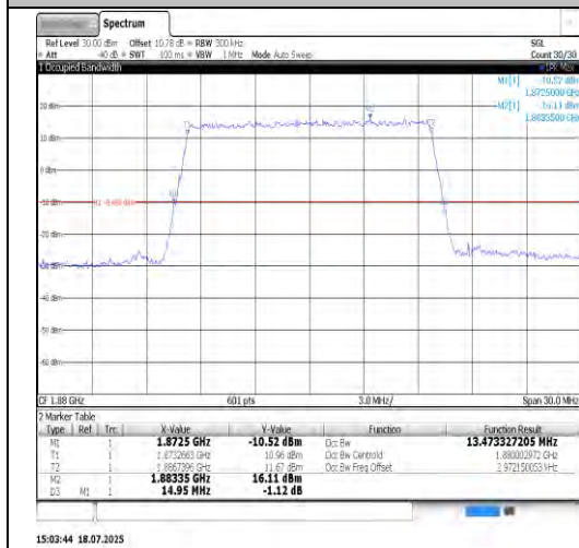
Band2-20MHz-QPSK-18900-100RB#0-PASS
