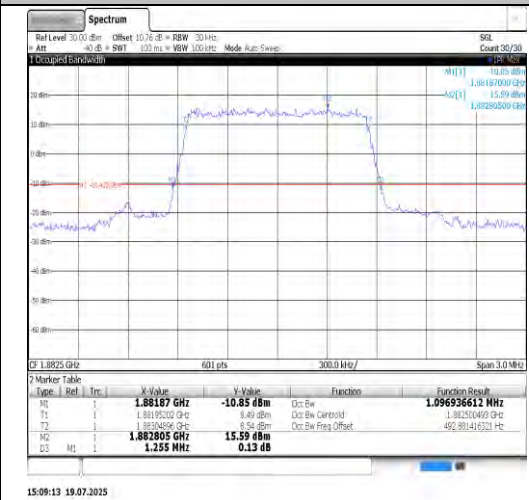
Band25-3MHz-QPSK-26365-15RB#0-PASS
