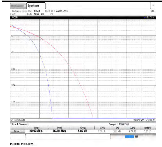
Band25-10MHz-QPSK-26365-50RB#0-PASS
