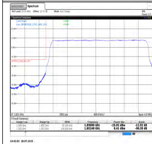
Band2-3MHz-QPSK-18615-15RB#14-PASS
