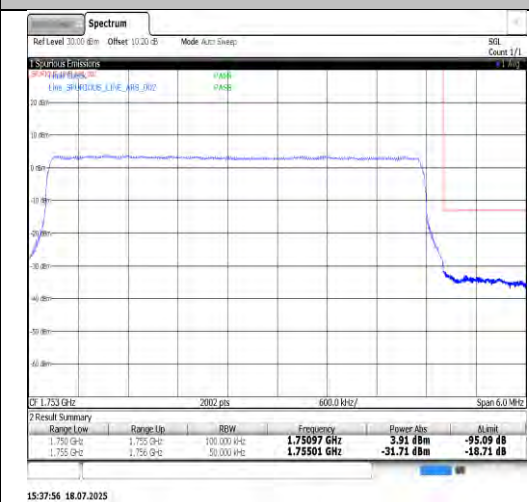
Band4-10MHz-QPSK-20000-1RB#49-PASS
