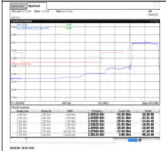
Band38-20MHz-QPSK-38150-1RB#99-PASS
