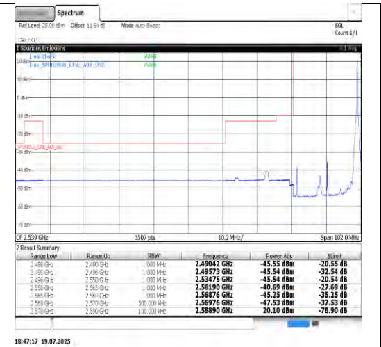
Band38-20MHz-QPSK-38150-1RB#0-PASS
