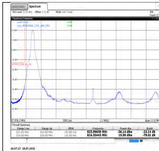
Band26(824-849)-10MHz-QPSK-26840-50RB#0-PASS
