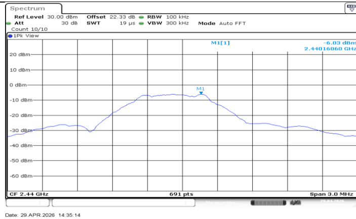
BLE 1M Ant1 2440 0~Reference
