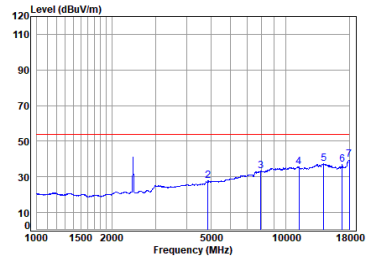
11g_TX_CH_06_Vertical-Avg
