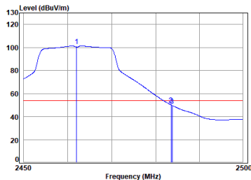
11g_TX_CH_11_Vertical-Avg
