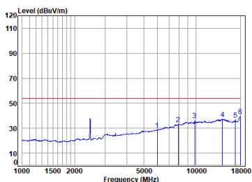
11g_TX_CH_11_Horizontal-Avg
