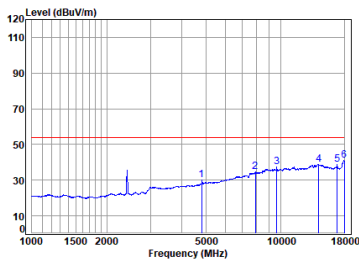
11n_20M_TX_CH_01_Horizontal-Avg
