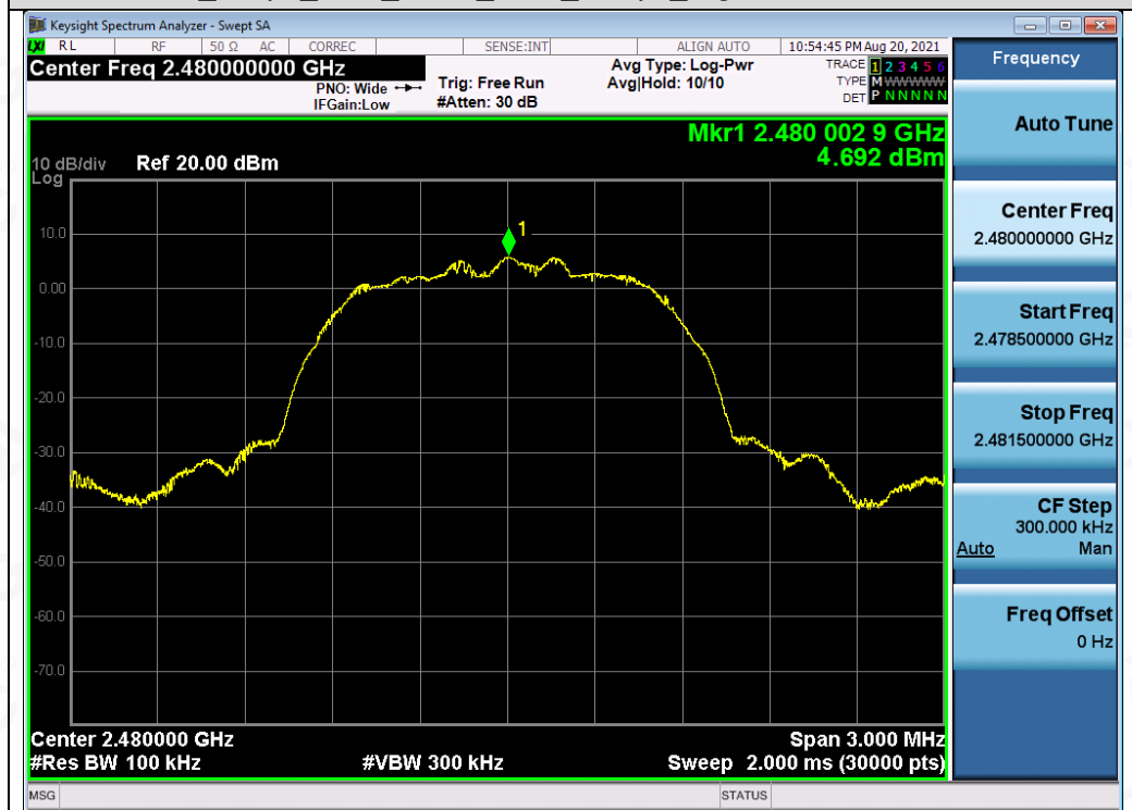
Test_Graph_EDR_ANT1_2480_2Mbps_Reference Level
