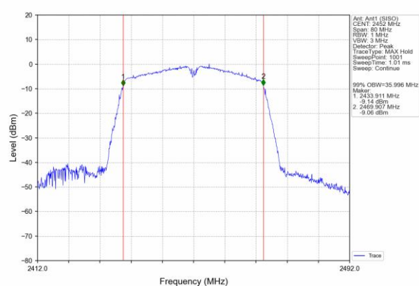
2452MHz
