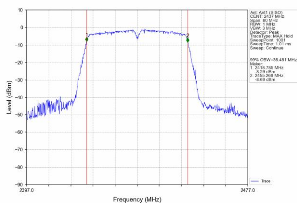
2437MHz
