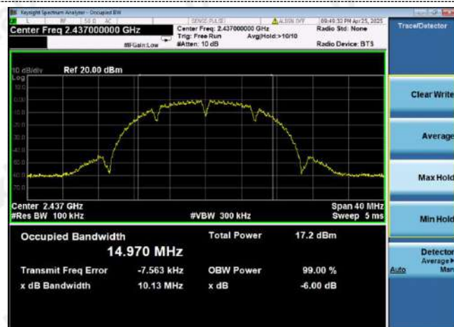
CH06
