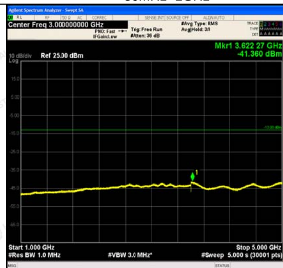
1GHz ~5GHz
