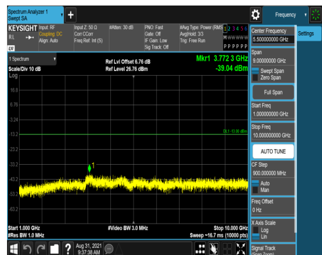
Band26-1.4MHz-QPSK-26797-1RB#0-Range2:1000~10000MHz
