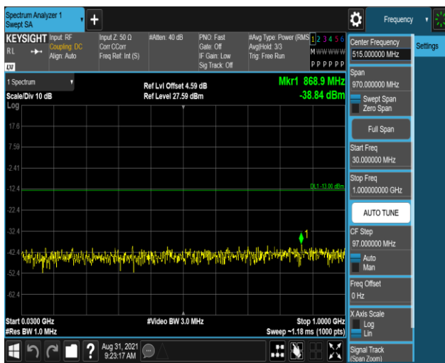
Band25-20MHz-QPSK-26365-1RB#0-Range1:30~1000MHz
