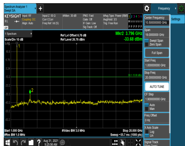
Band25-20MHz-16QAM-26590-1RB#0-Range2:1000~ 20000MHz
