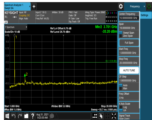
Band25-20MHz-QPSK-26365-1RB#0-Range2:1000~20000MHz
