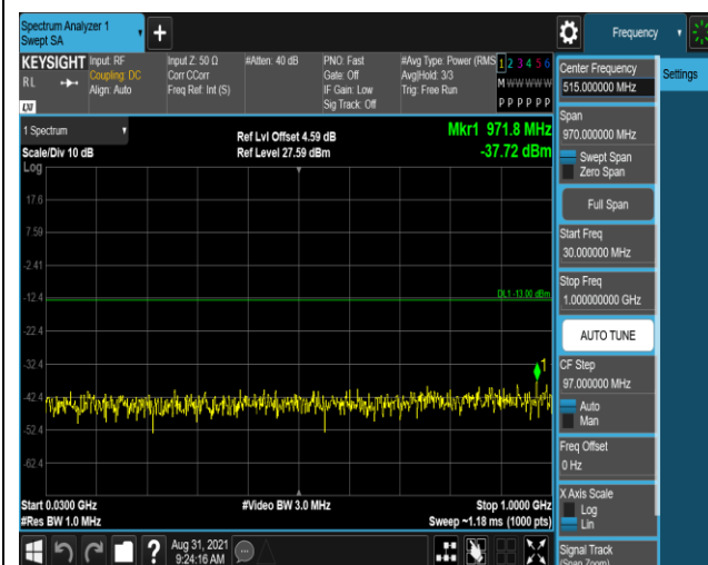
Band25-20MHz-QPSK-26365-1RB#0-Range1:30~1000MHz
