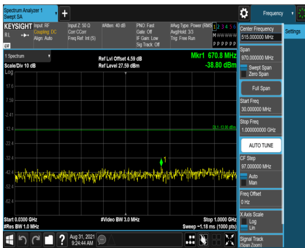
Band25-20MHz-16QAM-26590-1RB#0-Range1:30 ~1000MHz
