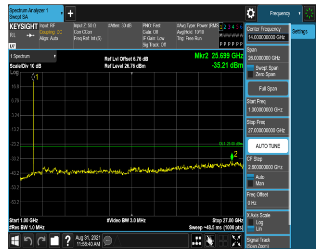
Band41-20MHz-QPSK-40640-1RB#0-Range2:1000~27000MHz
