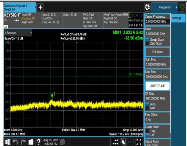
Band13-5MHz-QPSK-23255-1RB#0-Range2:1000~1 0000MHz
