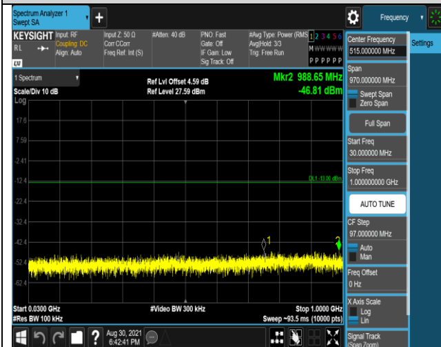
Band13-5MHz-QPSK-23255-1RB#0-Range1:30~100 0MHz
