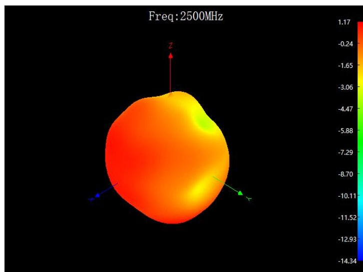
2500MHz 3D
