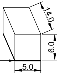
导电胶
