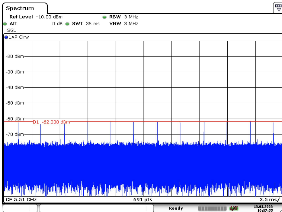
Radar Type 5 – 5510MHz
