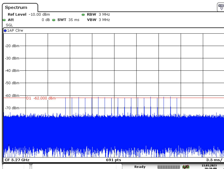
Radar Type 1A – 5270MHz
