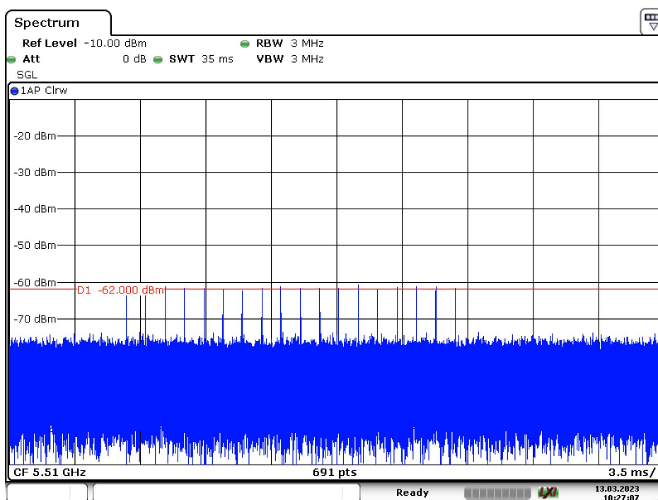
Radar Type 1A – 5510MHz
