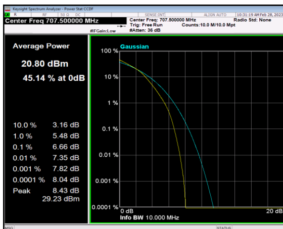
FDD12_MidRange_10MHz_707.5_fullIRB _Q16
