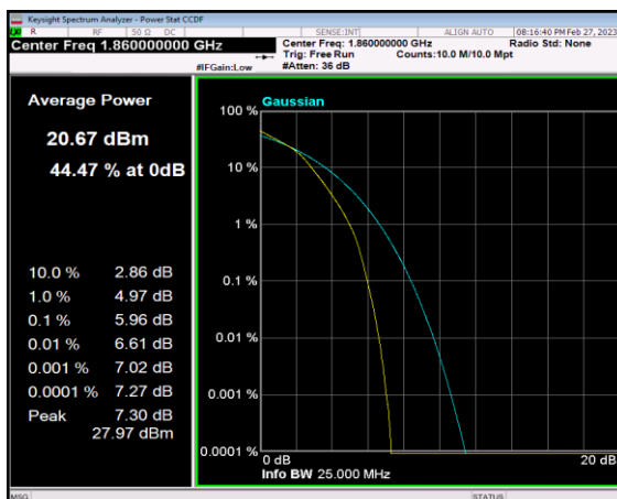
FDD25_LowRange_20MHz_1860_fullIRB _Q16
