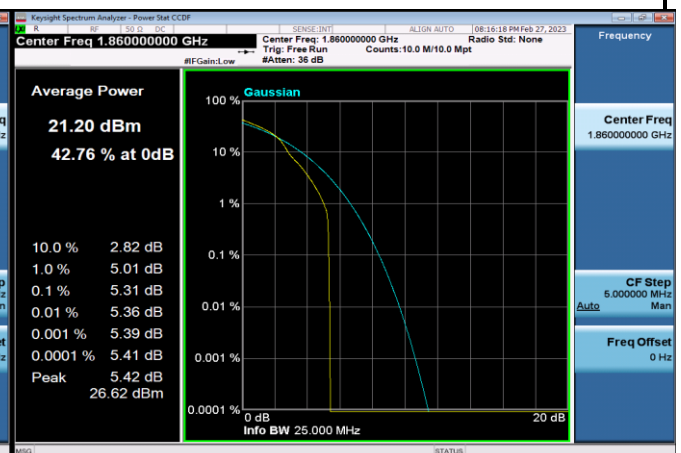
FDD25_LowRange_20MHz_1860_OneRB_high_Q16
