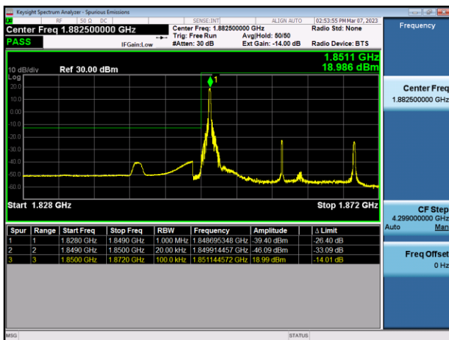
FDD25-20MHz-QPSK-LCH-1RB#0
