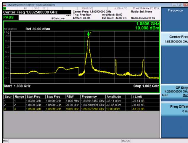
FDD25-10MHz-QPSK-LCH-50RB#0
