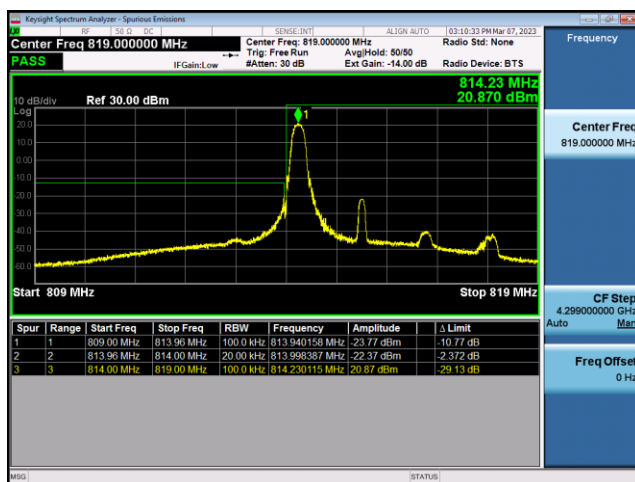
FDD26-Part 90-3MHz-QPSK-LCH-15RB#0
