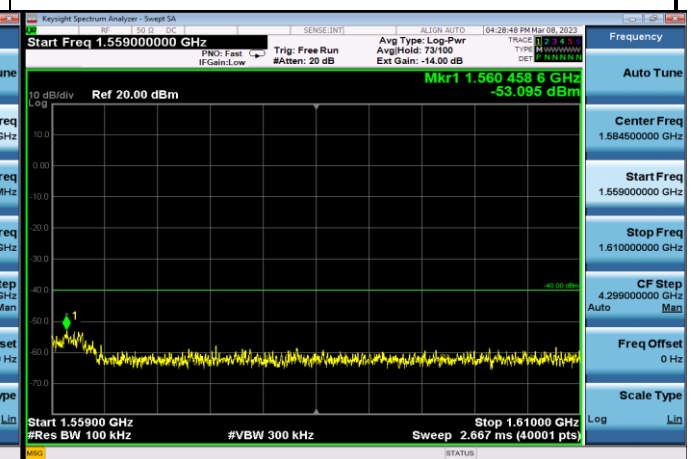
FDD13_HighRange_5MHz_1559MHz~1610MHz
