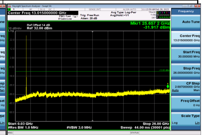
FDD25_HighRange_20MHz_30MHz~26GHz
