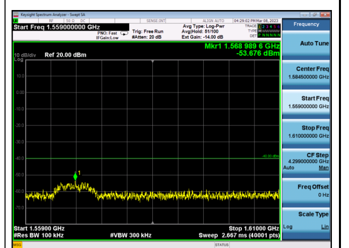
FDD13_HighRange_5MHz_1559MHz~1610MHz
