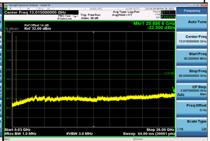
FDD13_HighRange_5MHz_30MHz~26GHz
