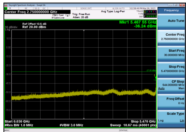
U-NII-2c ,Plot 2,30MHz~5470MHz-802.11 a(20MHz),5700MHz,Ant1
